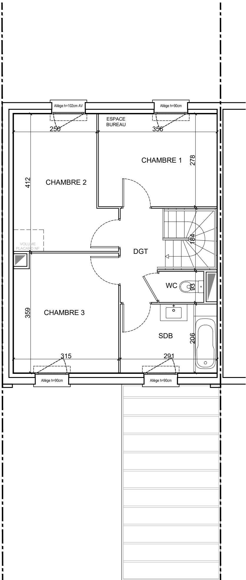
1ER ETAGE
