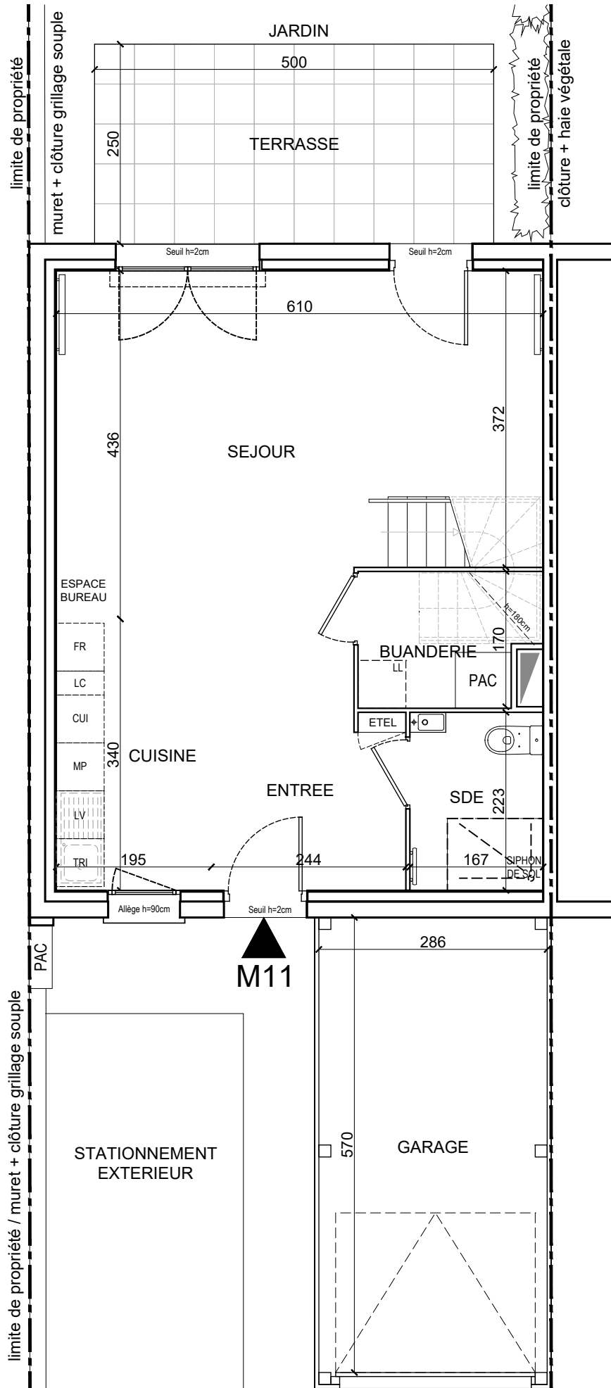
REZ-DE-JARDIN
