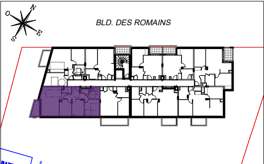
Appartement de 4 pièces n° 17 au 1er étage
