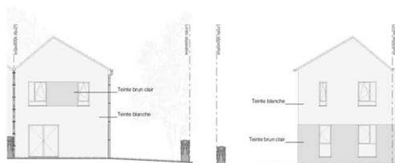
Façade Sud
