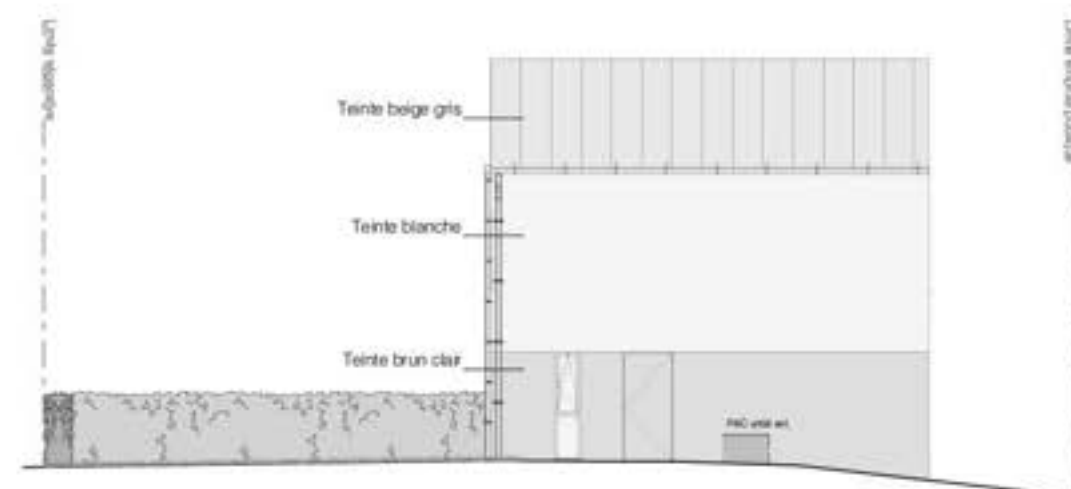
Façade Est
