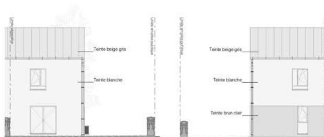
Façade Sud
