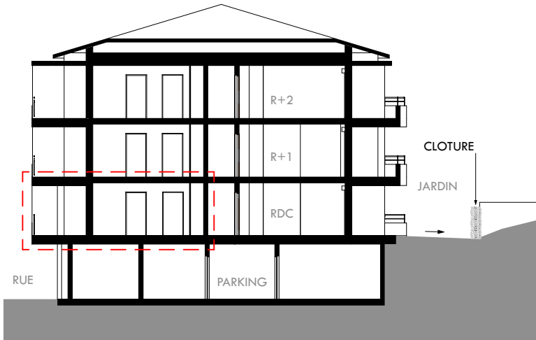
Coupe de principe sur rue
