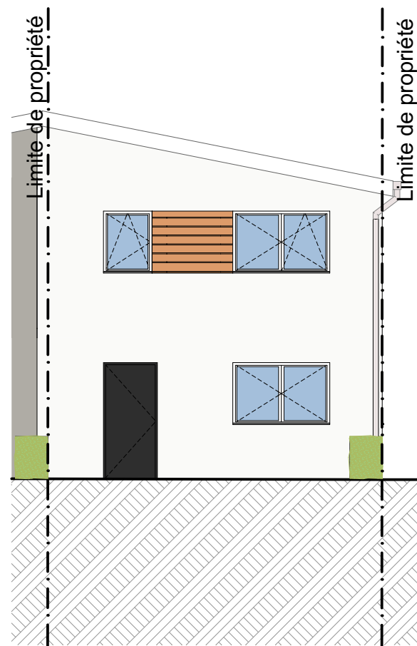
FACADE EST 1:100
