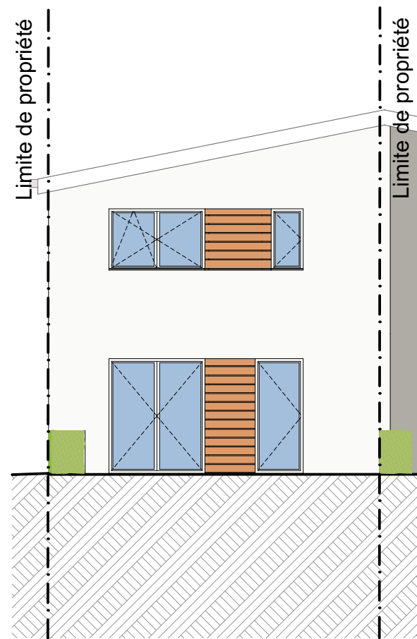
FACADE OUEST 1:100
