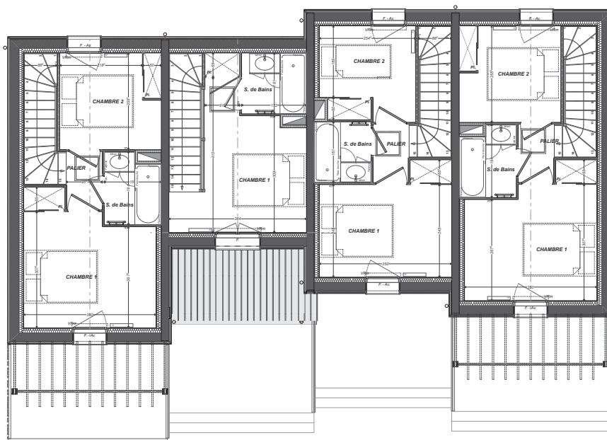
PLAN ETAGE
