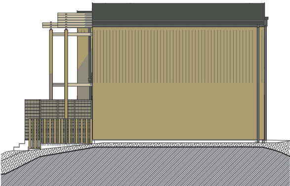
FACADE NORD
