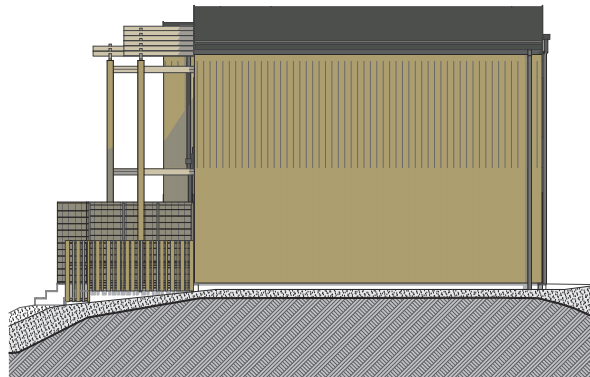
FACADE NORD
