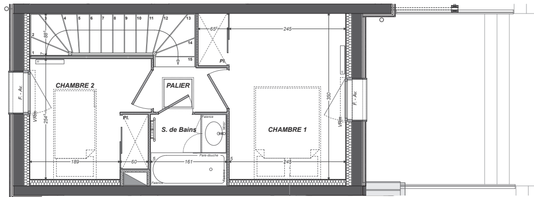
PLAN ETAGE
