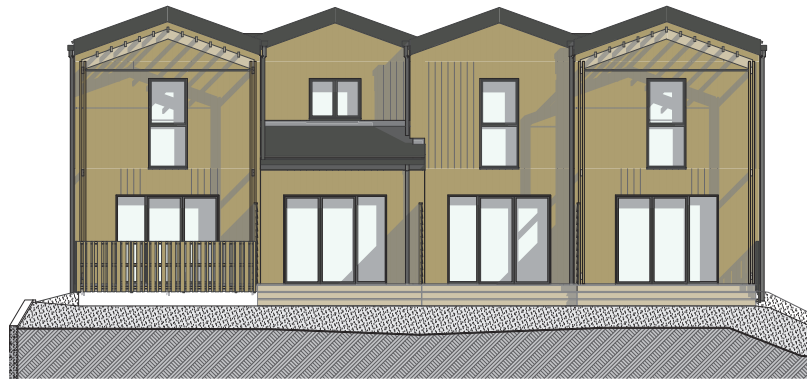
FACADE OUEST
