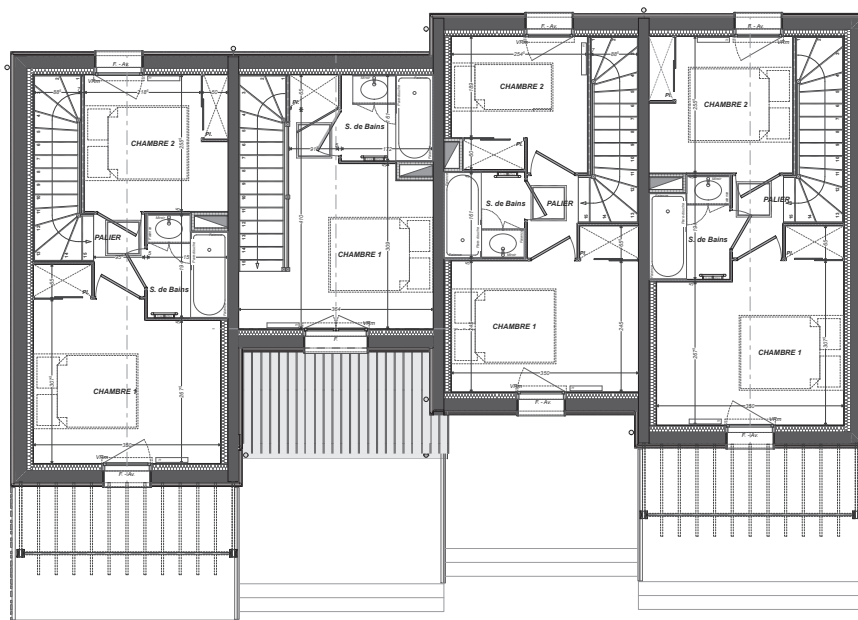
PLAN ETAGE
