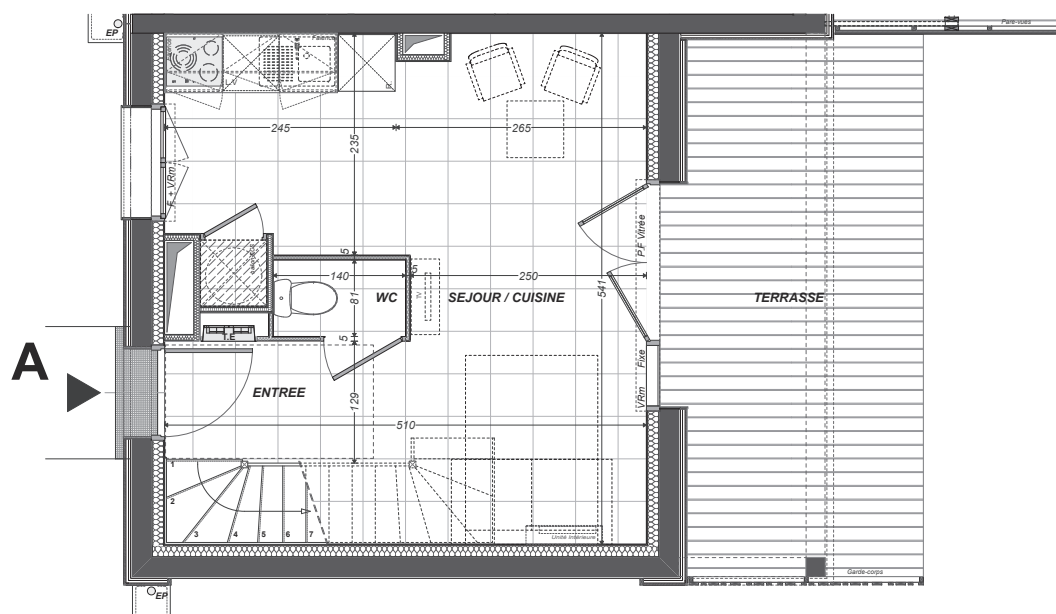
PLAN REZ DE CHAUSSEE
