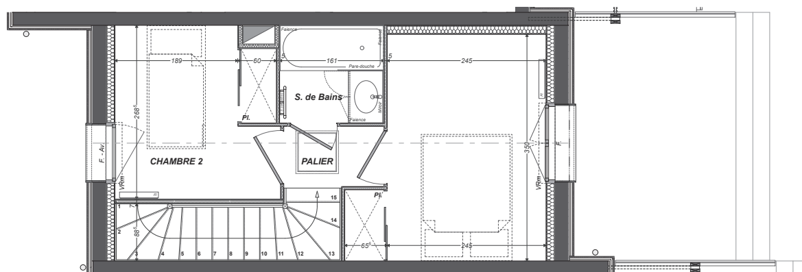
PLAN ETAGE
