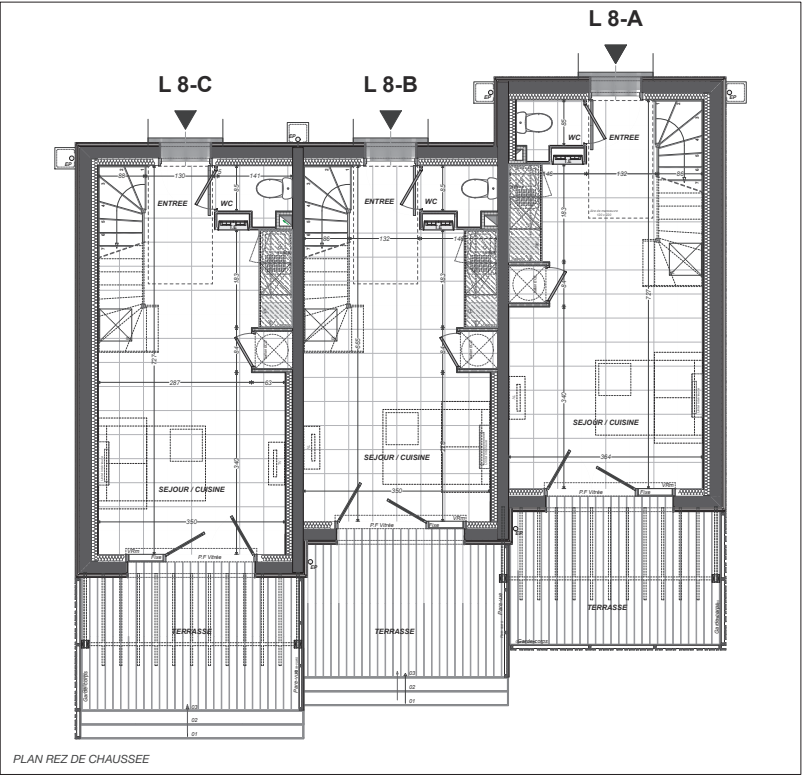
PLAN REZ DE CHAUSSEE
