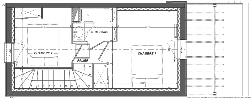
PLAN ETAGE
