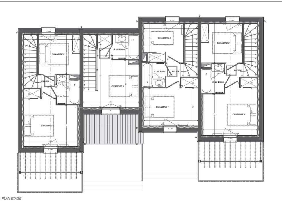
PLAN ETAGE
