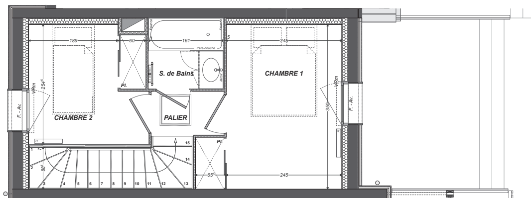
PLAN ETAGE
