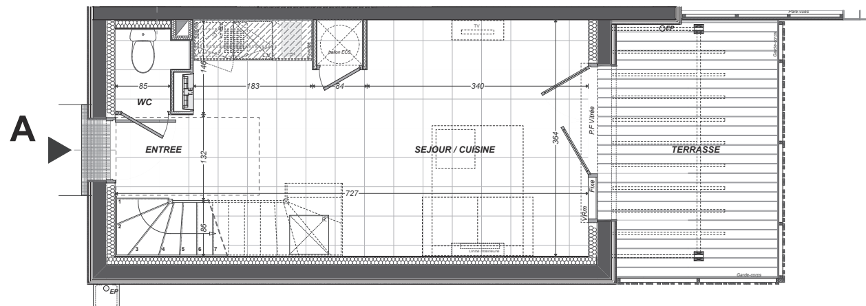
PLAN REZ DE CHAUSSEE
