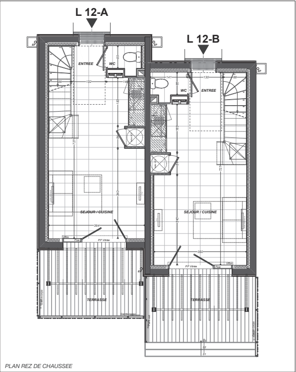
PLAN REZ DE CHAUSSEE
