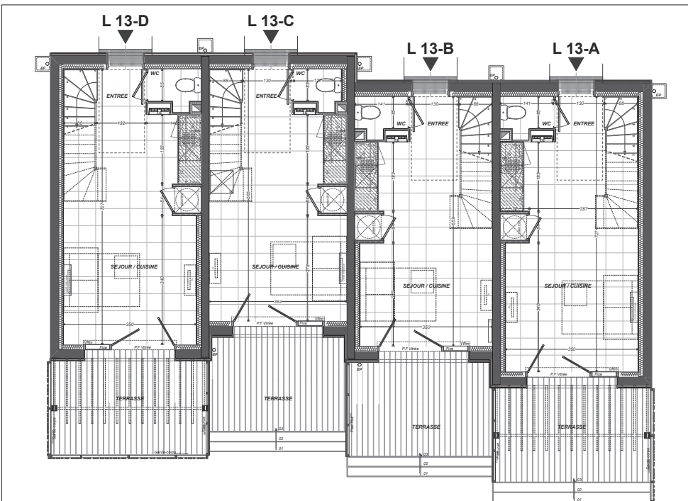
PLAN REZ DE CHAUSSEE
