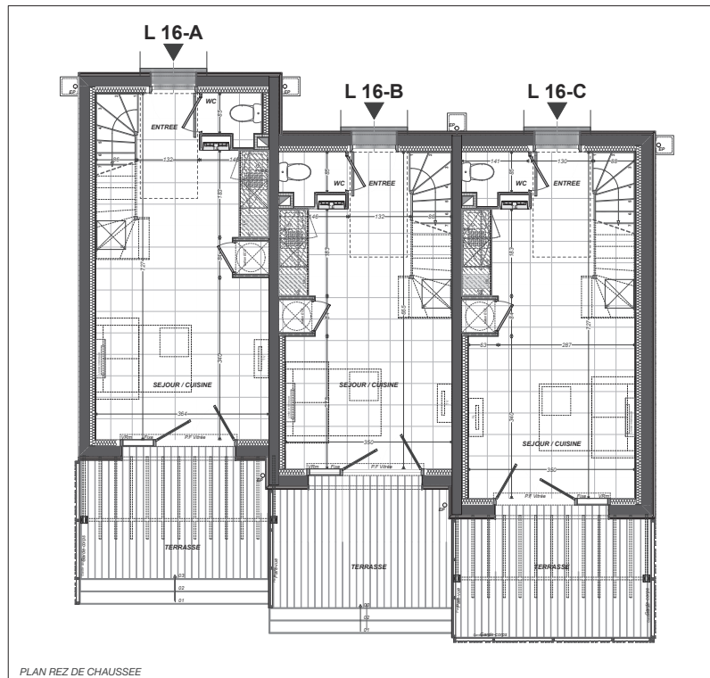
PLAN REZ DE CHAUSSEE
