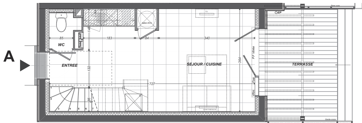
PLAN REZ DE CHAUSSEE
