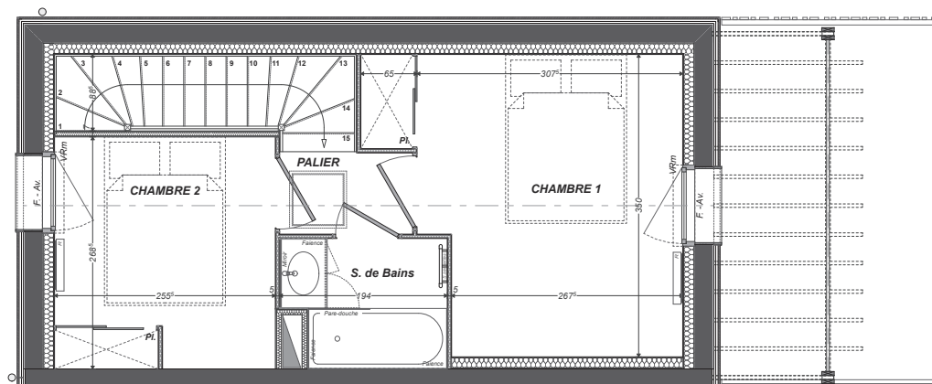
PLAN ETAGE
