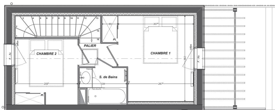
PLAN ETAGE
