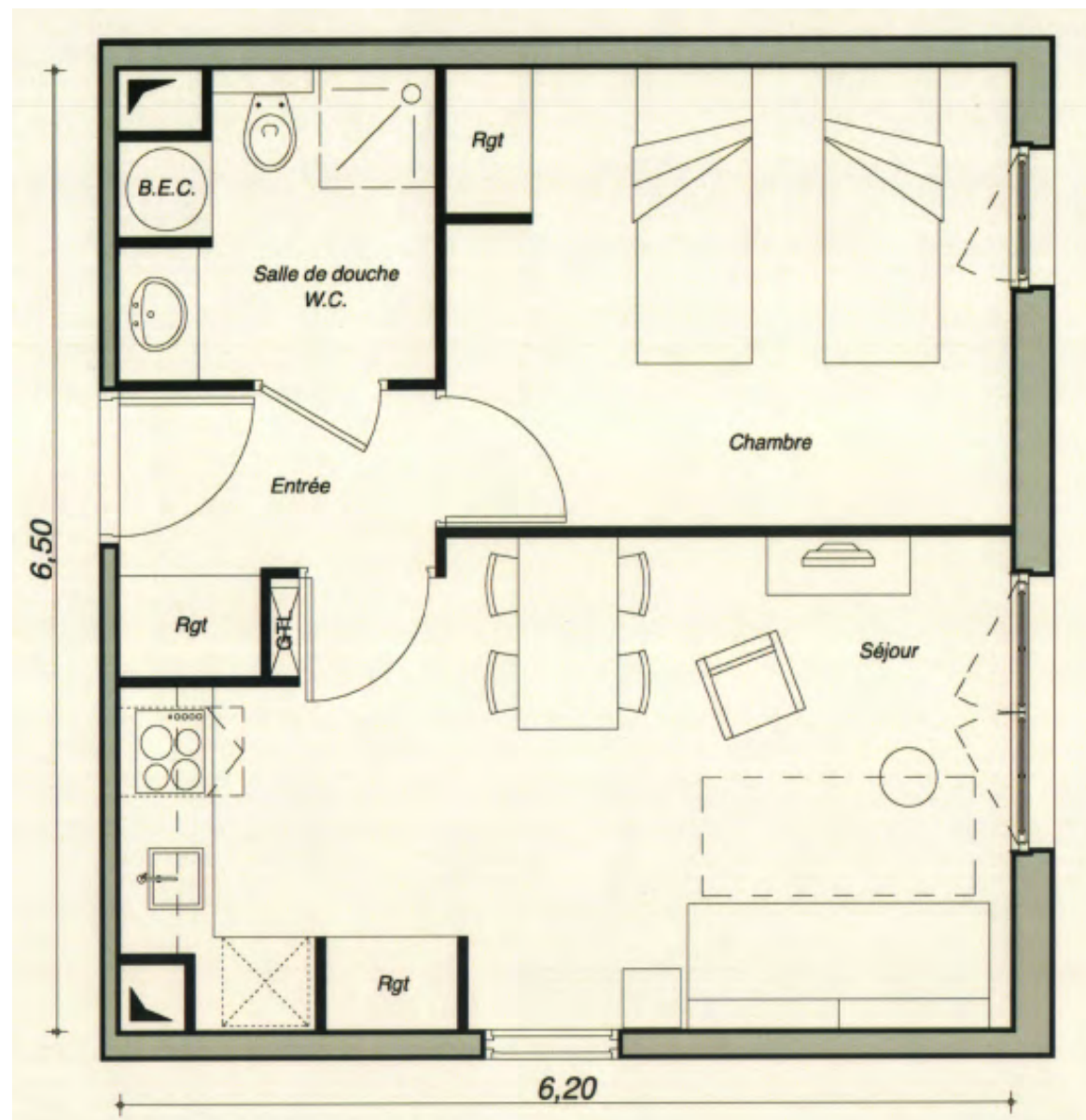
Schéma T2 - Lot n°128 - R+1
