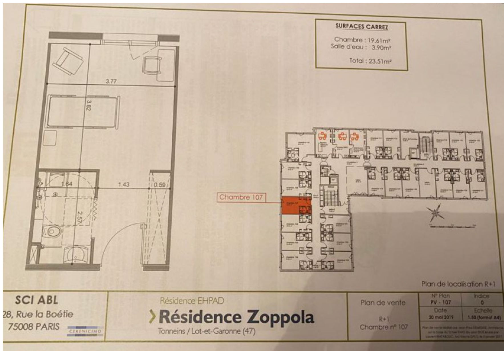
Plan Chambre simple - Lot n°107 - R+1
