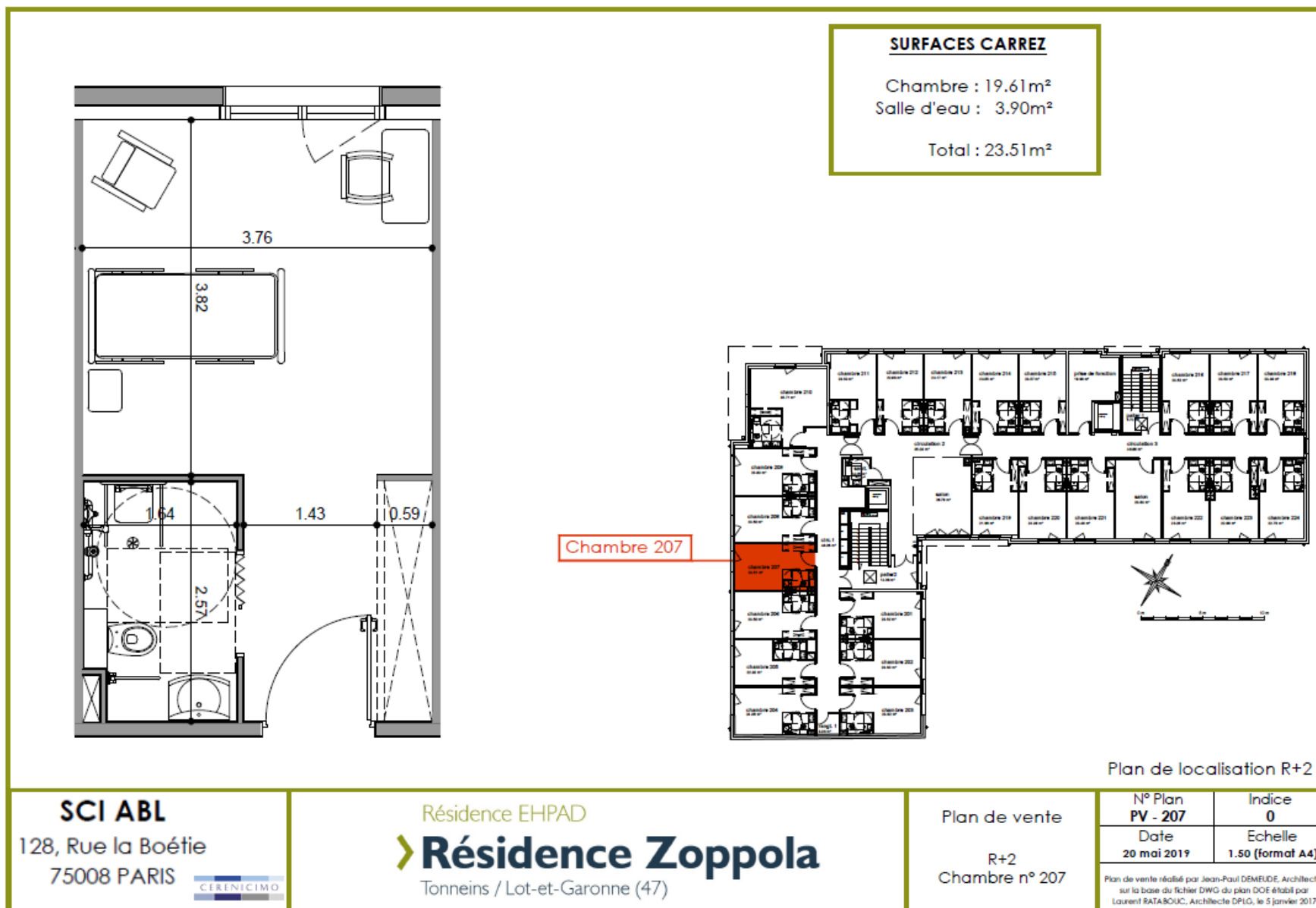
Plan Chambre simple - Lot n° 207 - R+2
