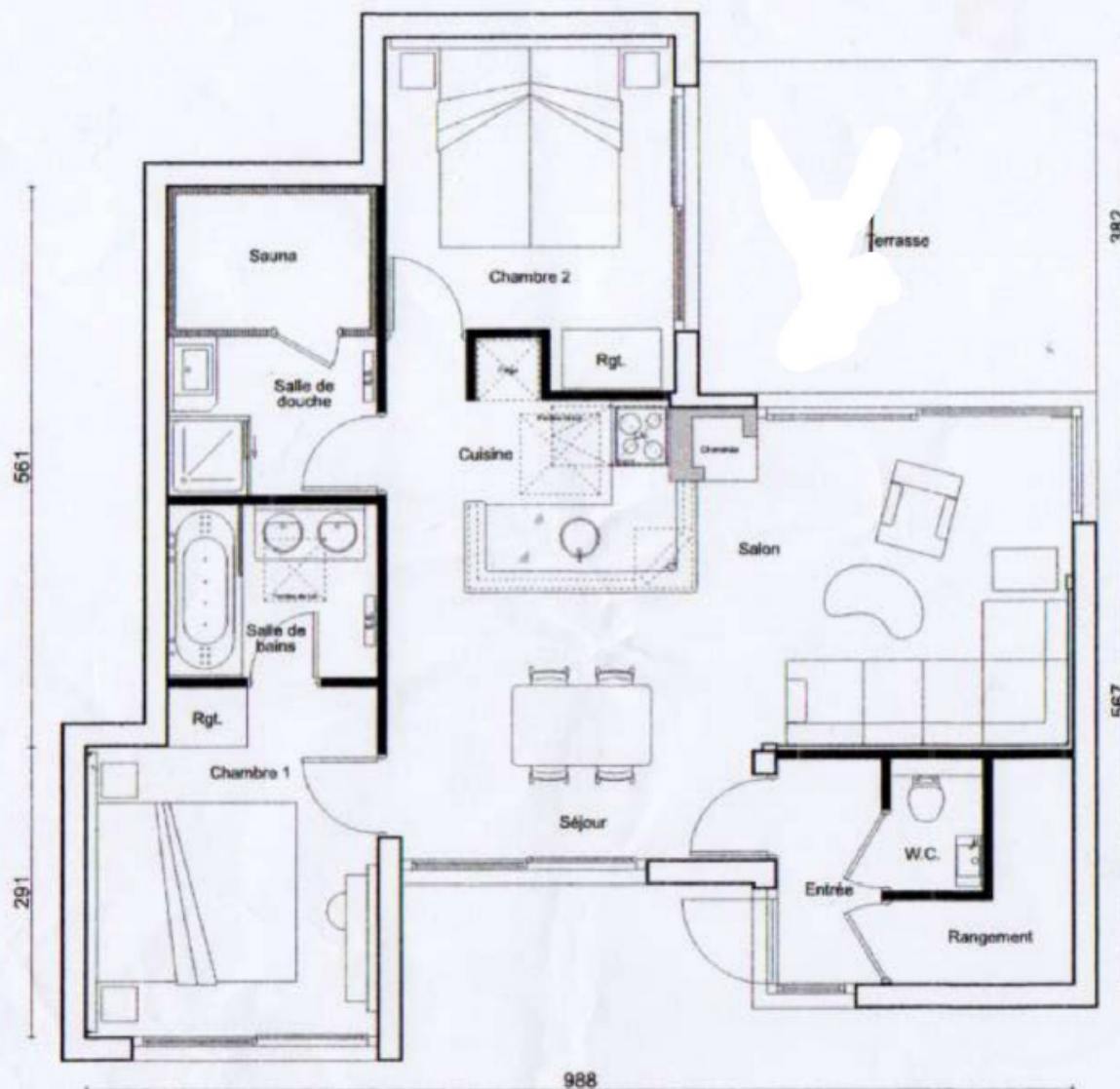
Plan Maison T3 - Lot n° 65-03 - RDC
