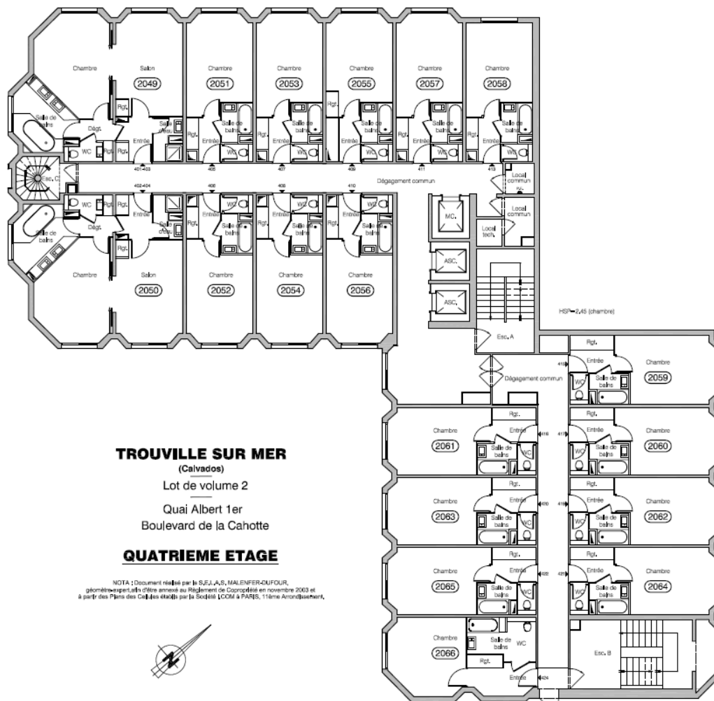
Plan Etage - R+4
