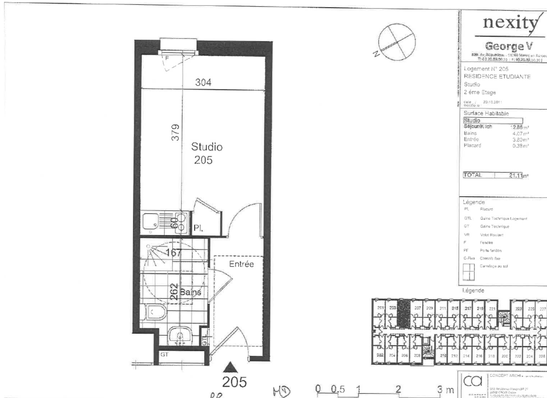
Plan Studio - Lot n° 205 - R+2
