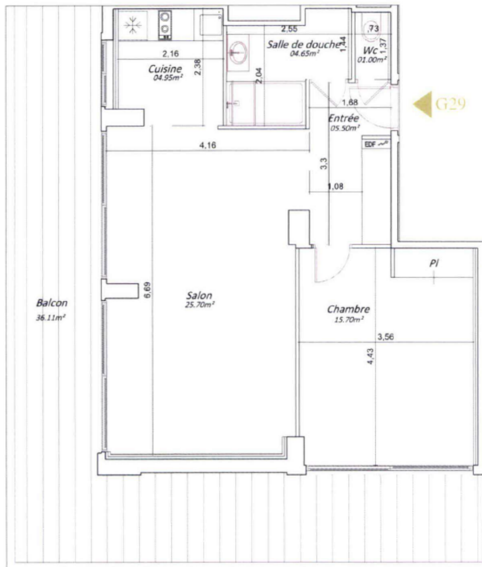
Plan T2 - Lot n° G29 - R+2
