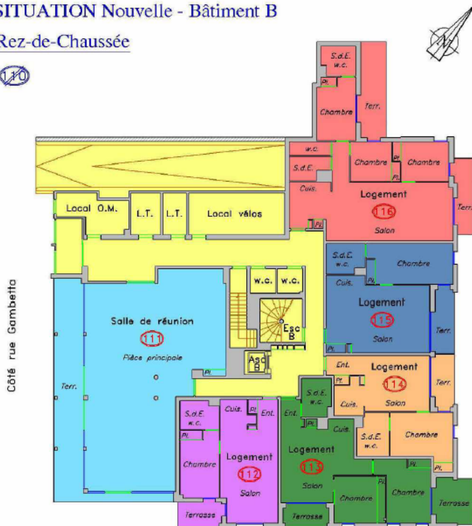
Plan Etage RDC– Lot n°116
