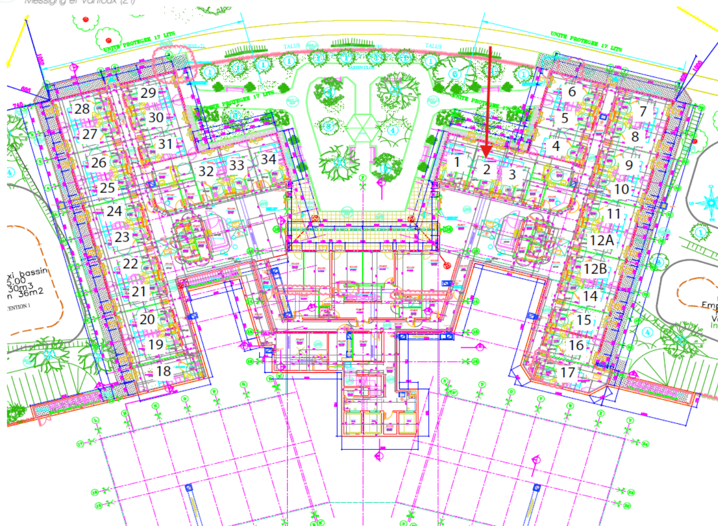
Plan Etage RDJ
