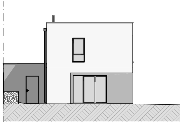
Façade Ouest
