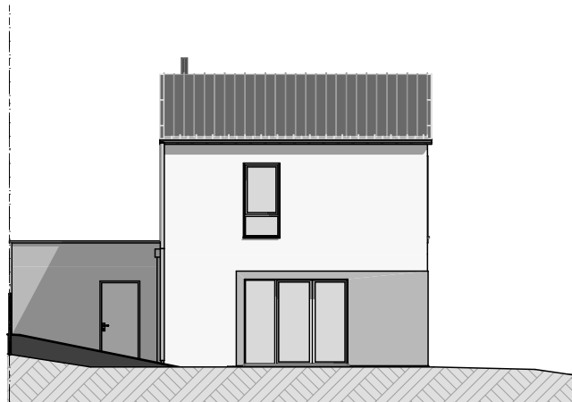
Façade Ouest
