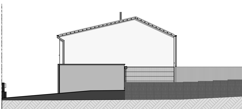
Façade Nord
