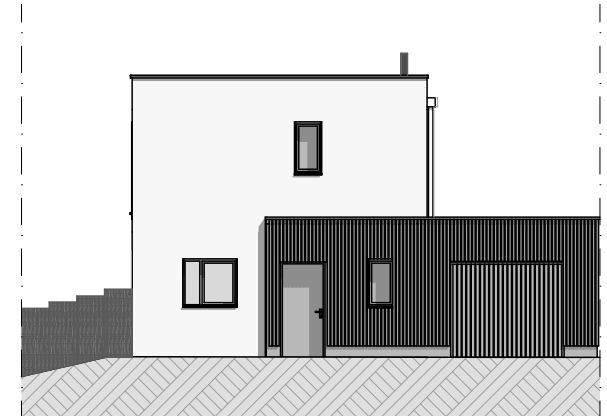
Façade Est
