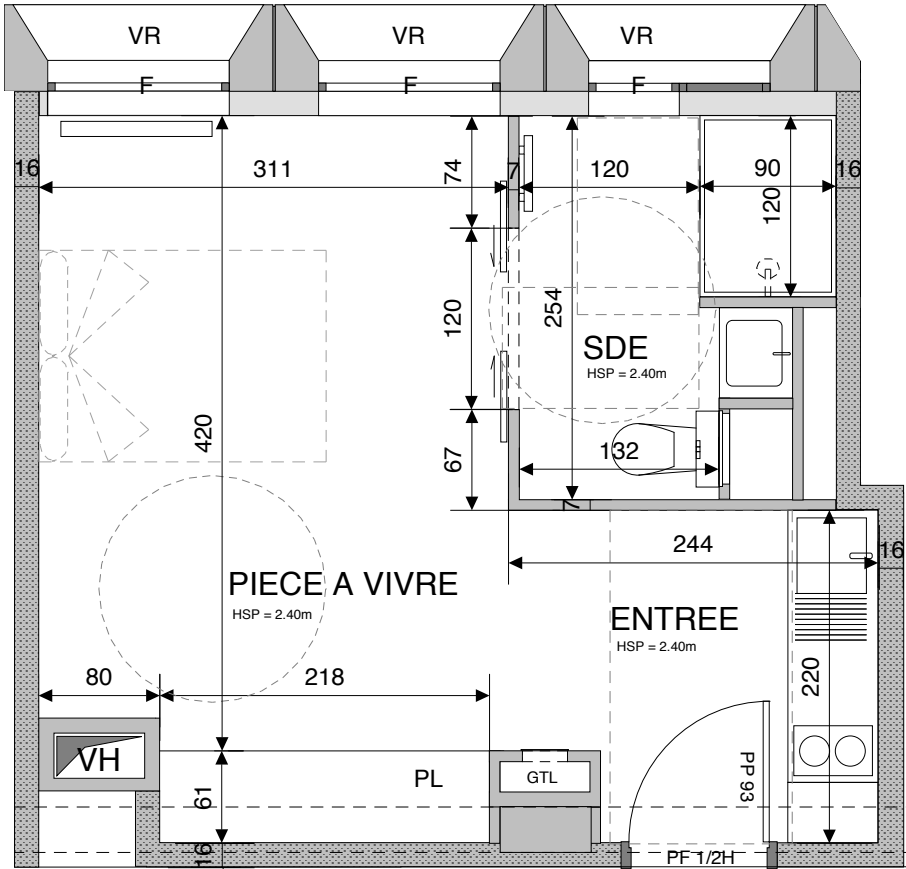
Lgt. 14 23,75 m2
