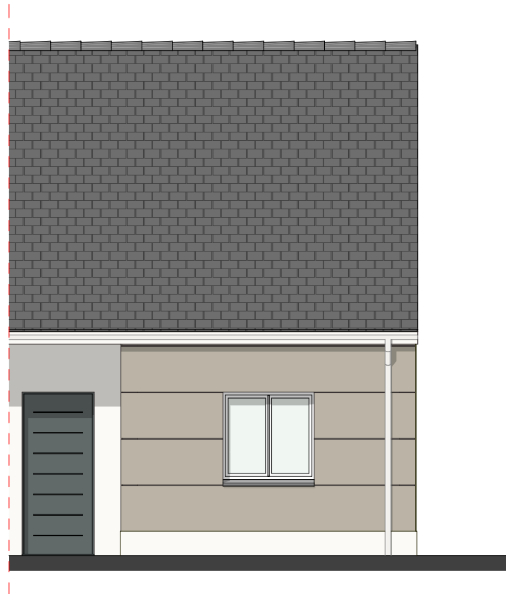
Façade entrée
