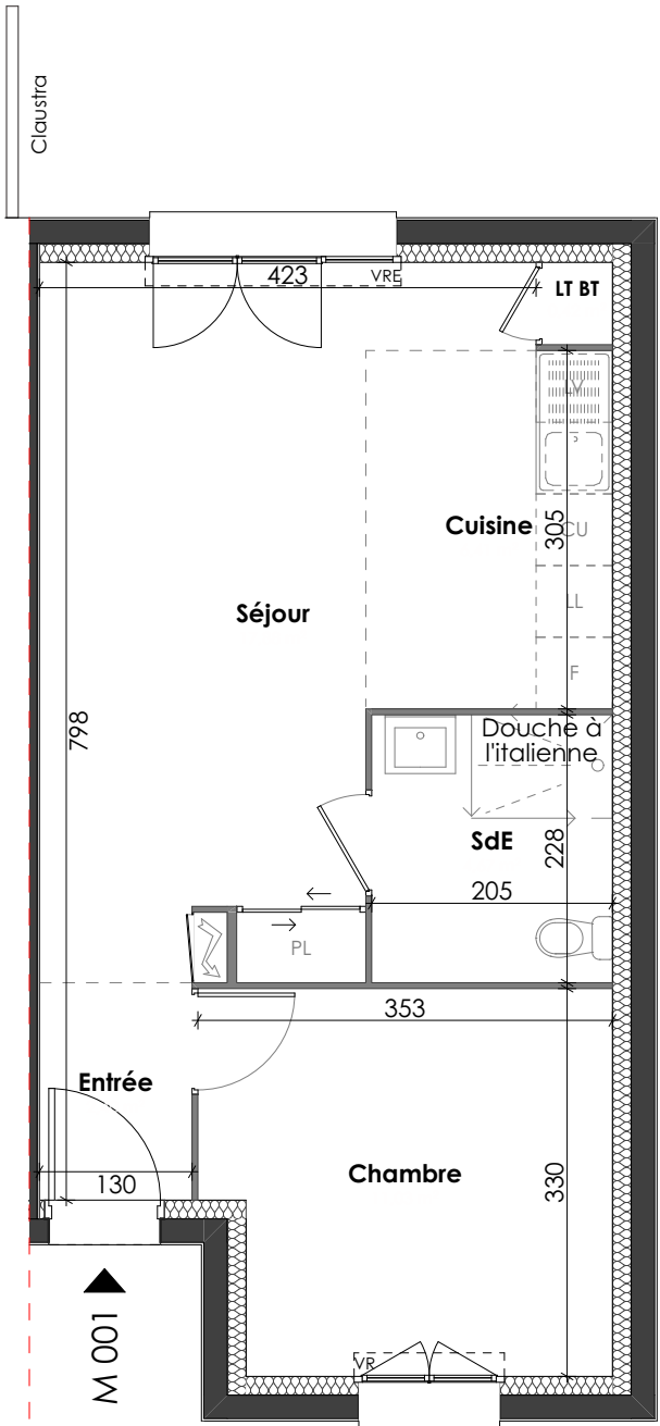
Rez-de-chaussée
