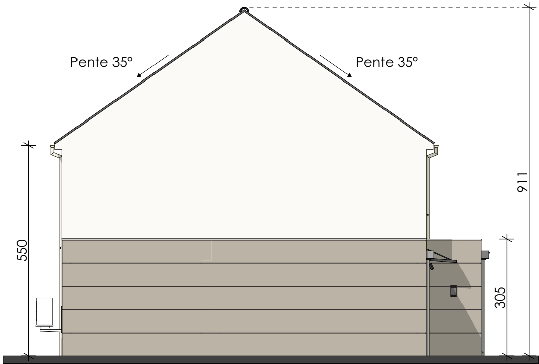
Pignon gauche
