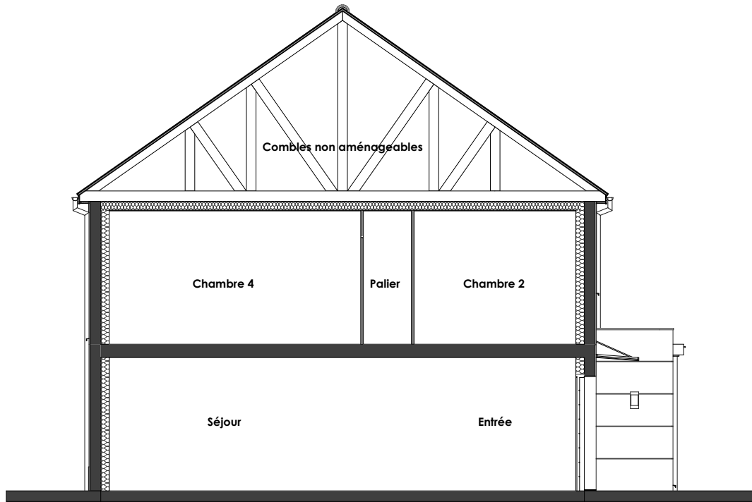
Coupe
