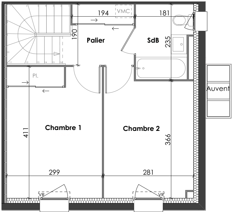
Etage
