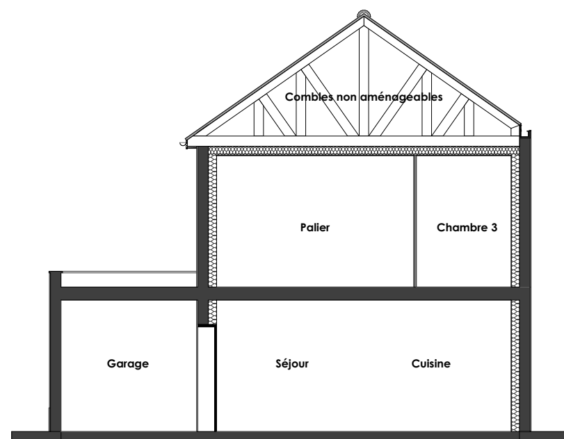
Coupe
