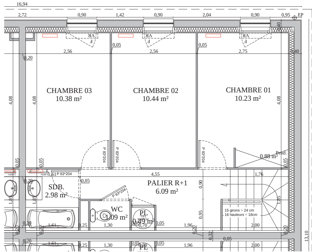
PLAN DE NIVEAU ETAGE - Ech : 1/50e
