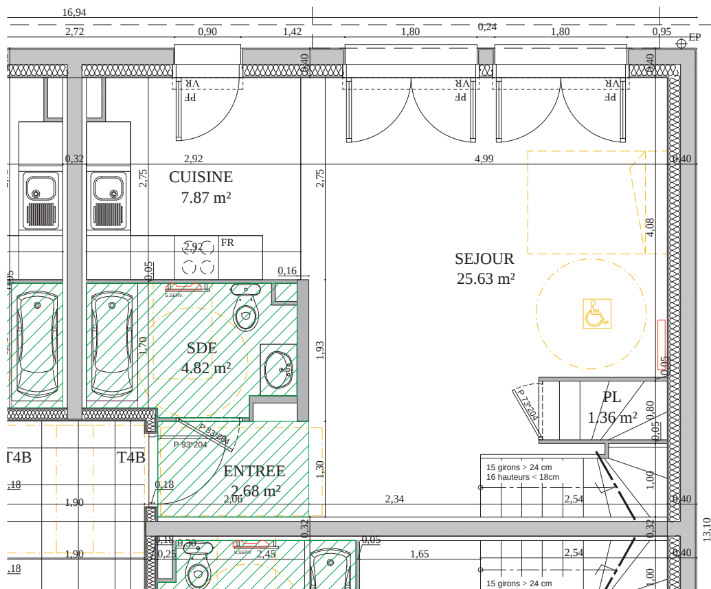
PLAN DE NIVEAU RDC PMR - Ech : 1/50e
