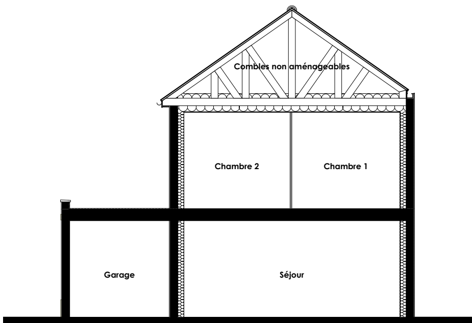
Coupe
