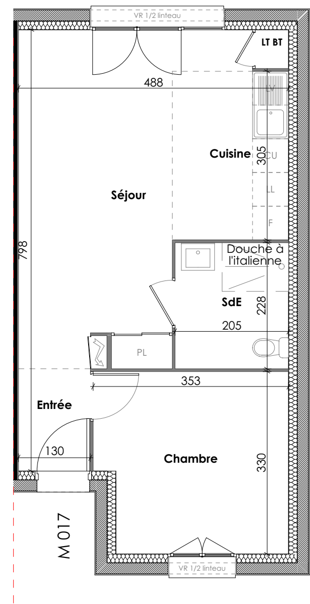
Rez-de-chaussée
