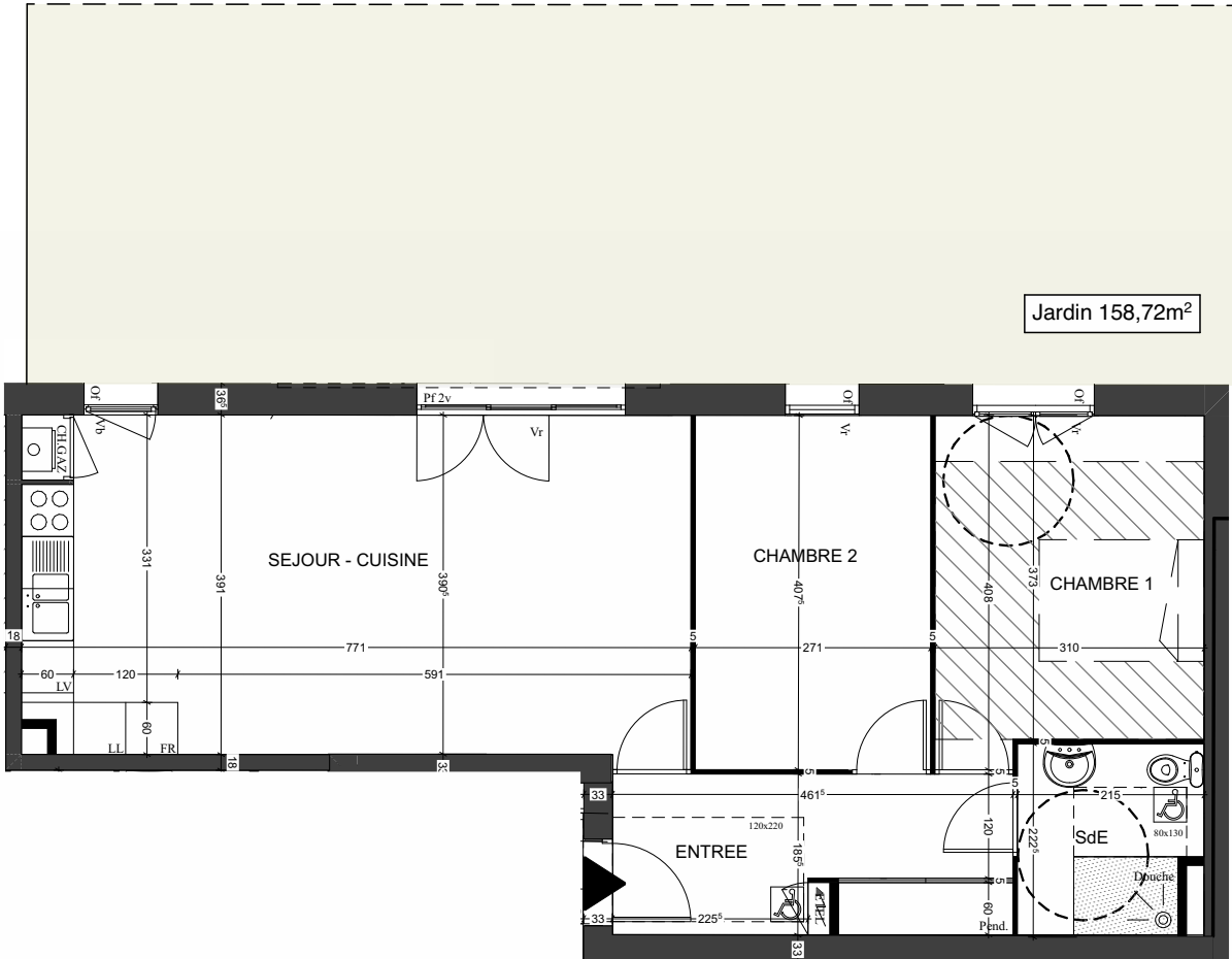
Plans du bâtiment
