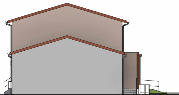
FACADE GAUCHE - Façade du pignon du garage accolée à la façade du pignon voisin
