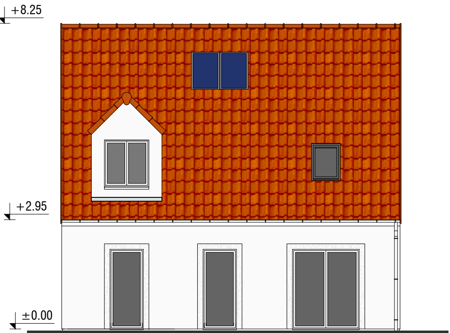
FAÇADE ARRIÈRE
