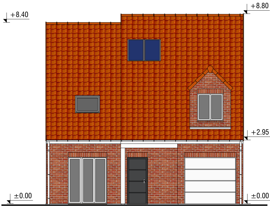
FAÇADE AVANT
