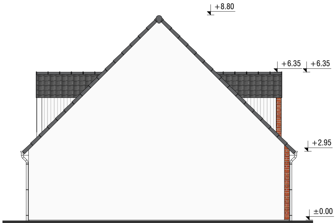
PIGNON GAUCHE
