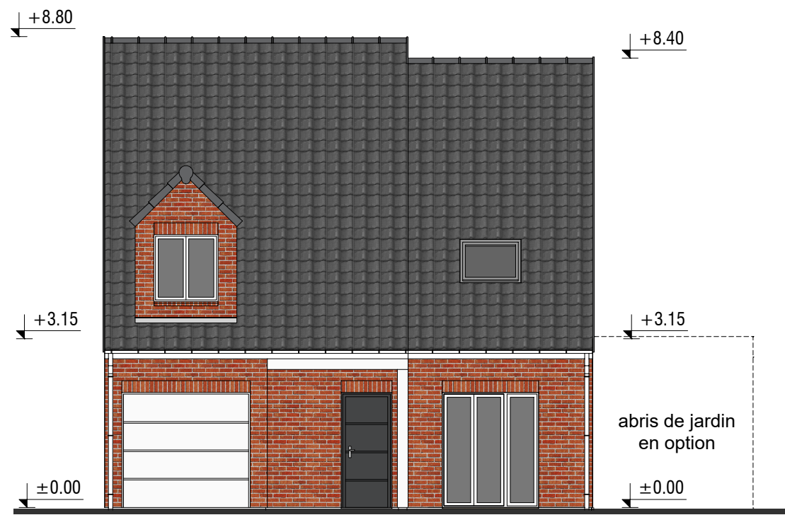
FAÇADE AVANT
