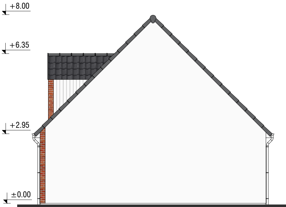
PIGNON DROIT
