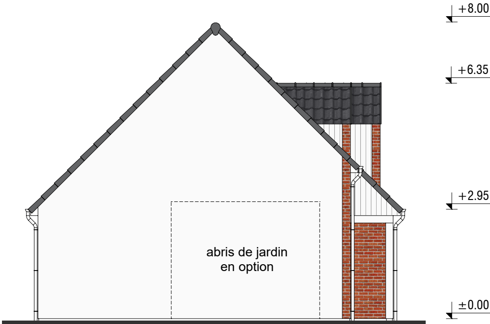
PIGNON GAUCHE
