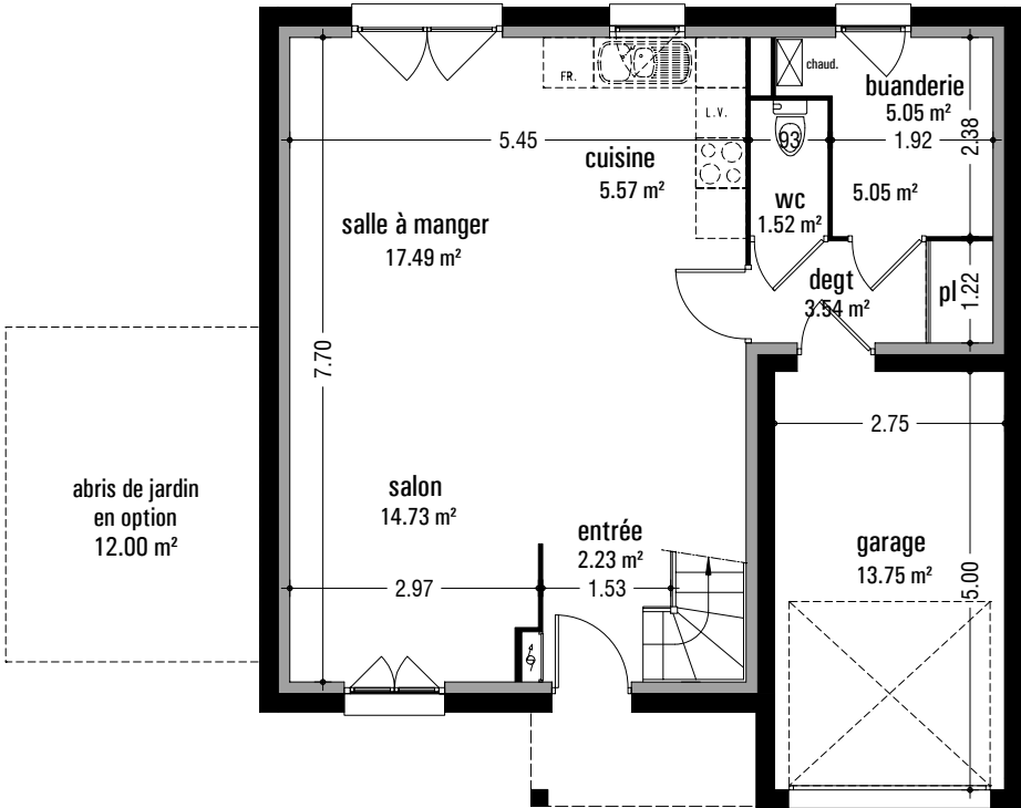
rez-de-chaussée
