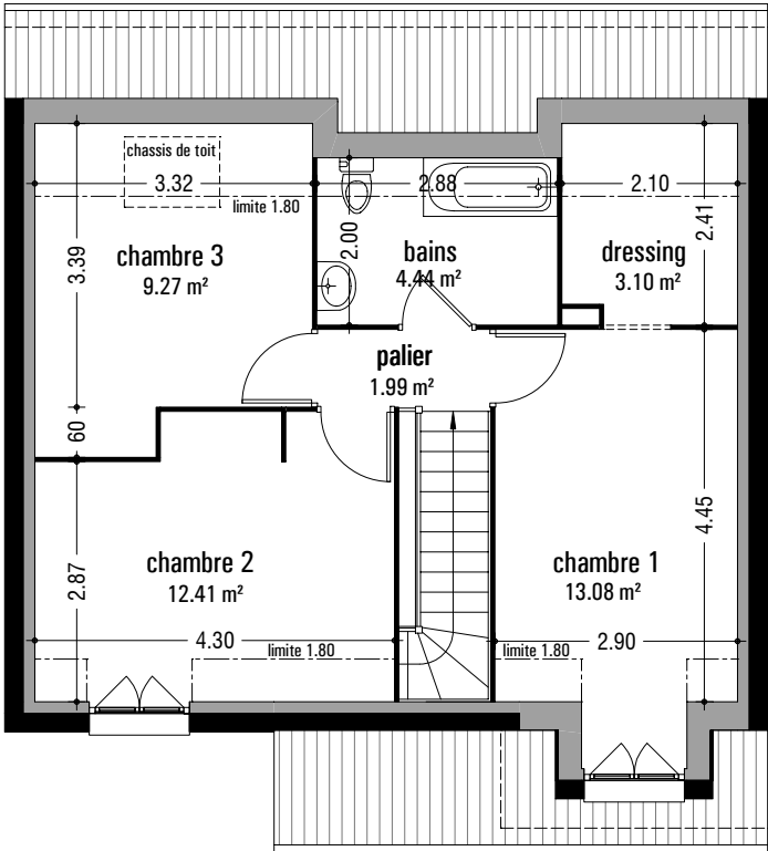
étage
