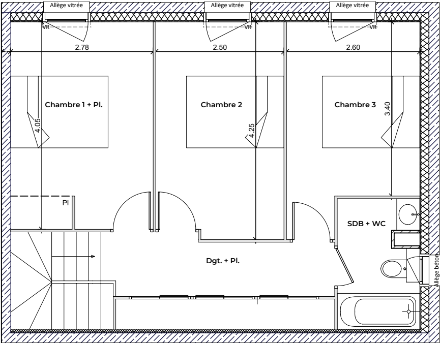
Plan d'étage
