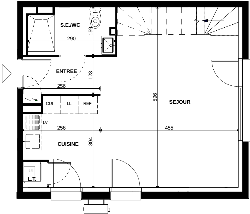
REZ DE CHAUSSEE
