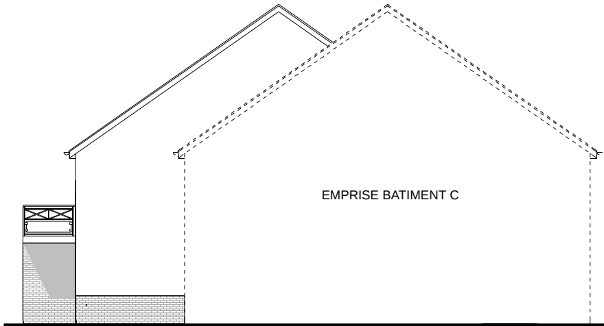
PIGNON DROIT
