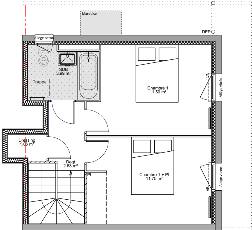
Plan d'étage
